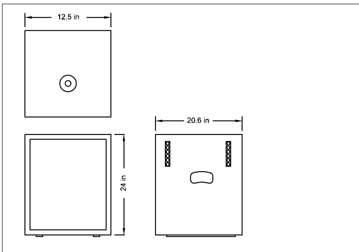
DIMENSIONS: 520mm(W) x 513mm(D) x 610mm(H)
